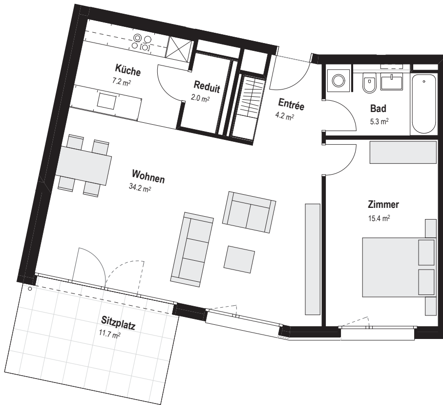
ERDGESCHOSS
