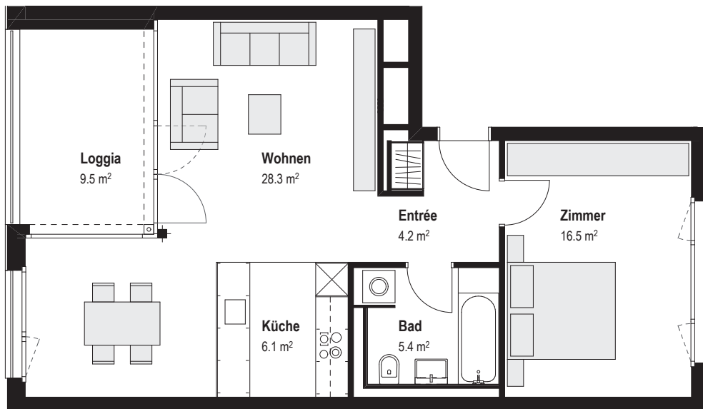
1.OG – 3.OG
