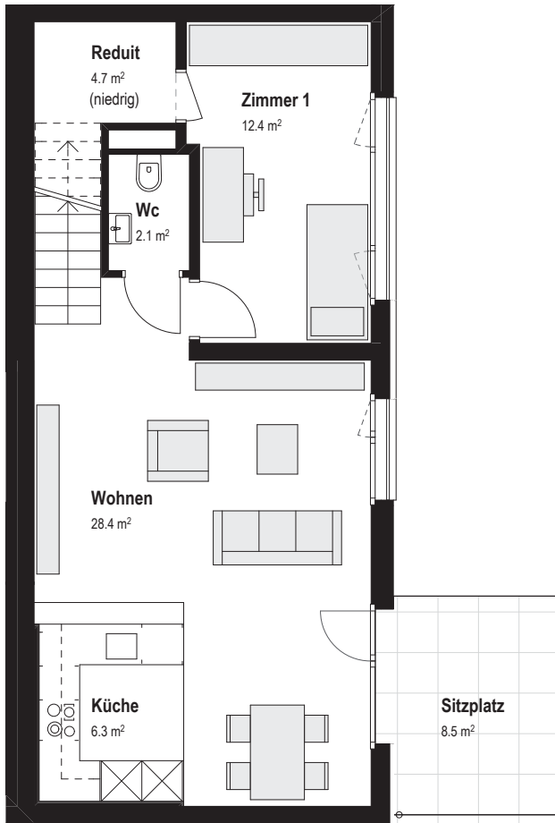
HOFGESCHOSS
